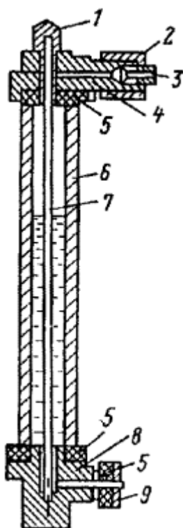
Рис. 4. Маслоуказатель маслонаполненного ввода напряжением 110 кВ.
