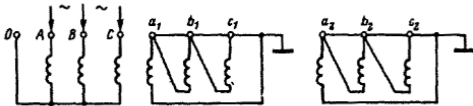
Рис. 23. Схема контрольного прогрева трансформатора токами короткого замыкания.
