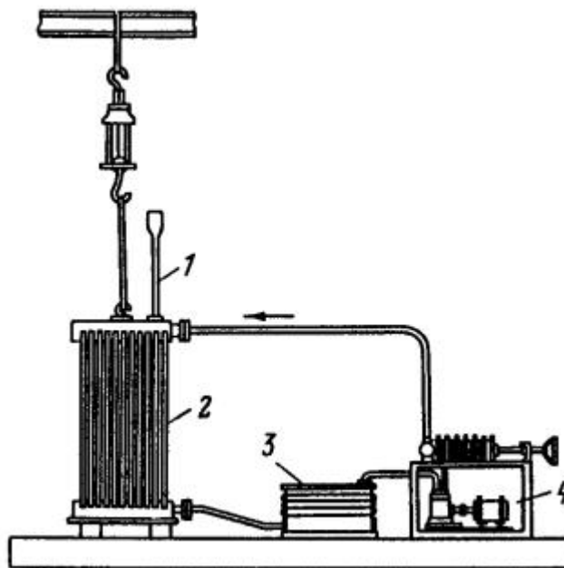
Рис. 8. Промывка радиатора.
