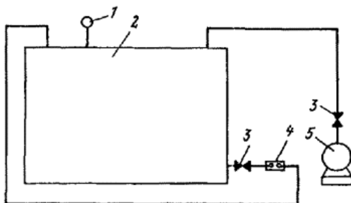
Рис. 22. Схема контрольной подсушки.
