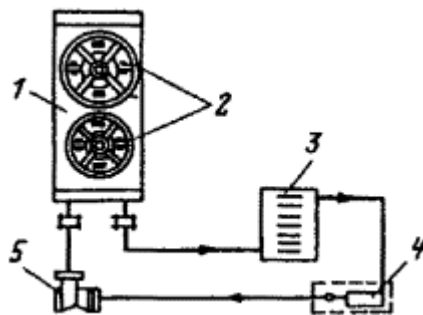
Рис. 21. Принципиальная схема промывки маслоохладительного устройства.
