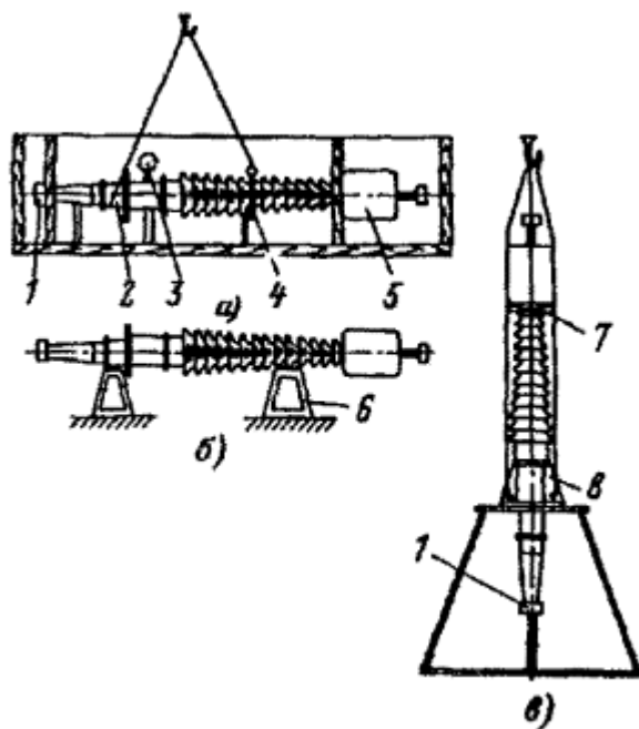
Рис. 5. Распаковка маслонаполненного герметичного ввода напряжением 110 кВ.
