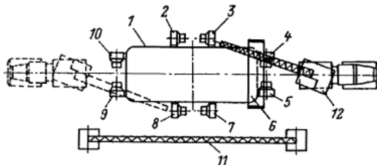
Рис. 20. Монтаж элементов навесной маслоохладительной системы ДЦ.
