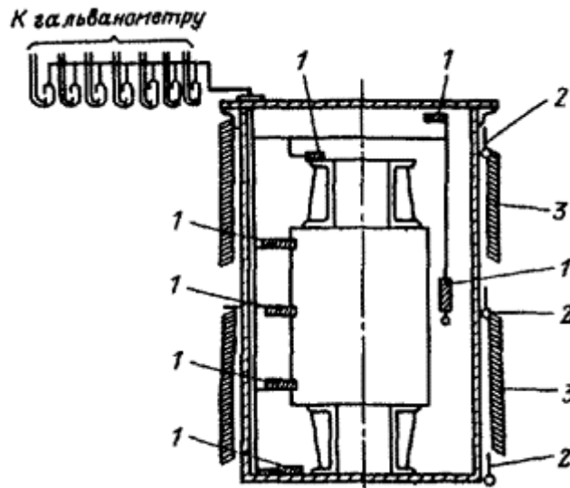
Рис. 28. Установка термопар и термометров при сушке трансформаторов.
