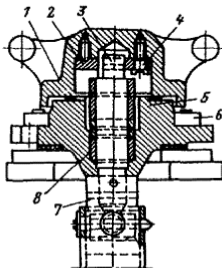
Рис. 14. Привод переключателей барабанного типа.
