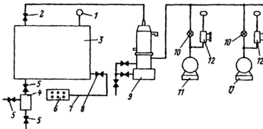
Рис. 29. Схема сушки трансформатора.
