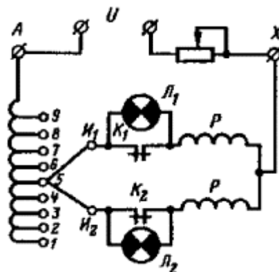
Рис. 16. Схема снятия круговой диаграммы переключающего устройства.
