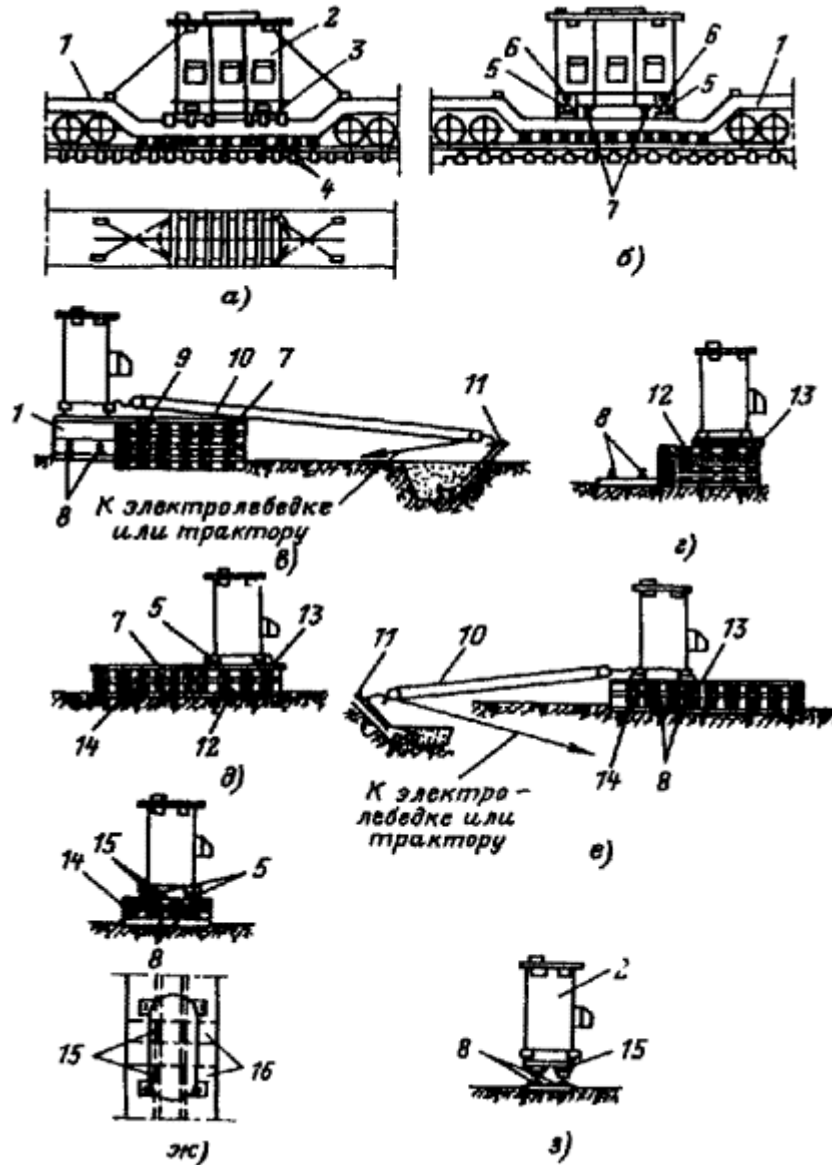
Рис. 1. Схема последовательности разгрузки трансформатора гидравлическими домкратами.
