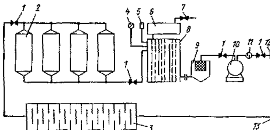
Схема установки для очистки трансформаторного масла.
