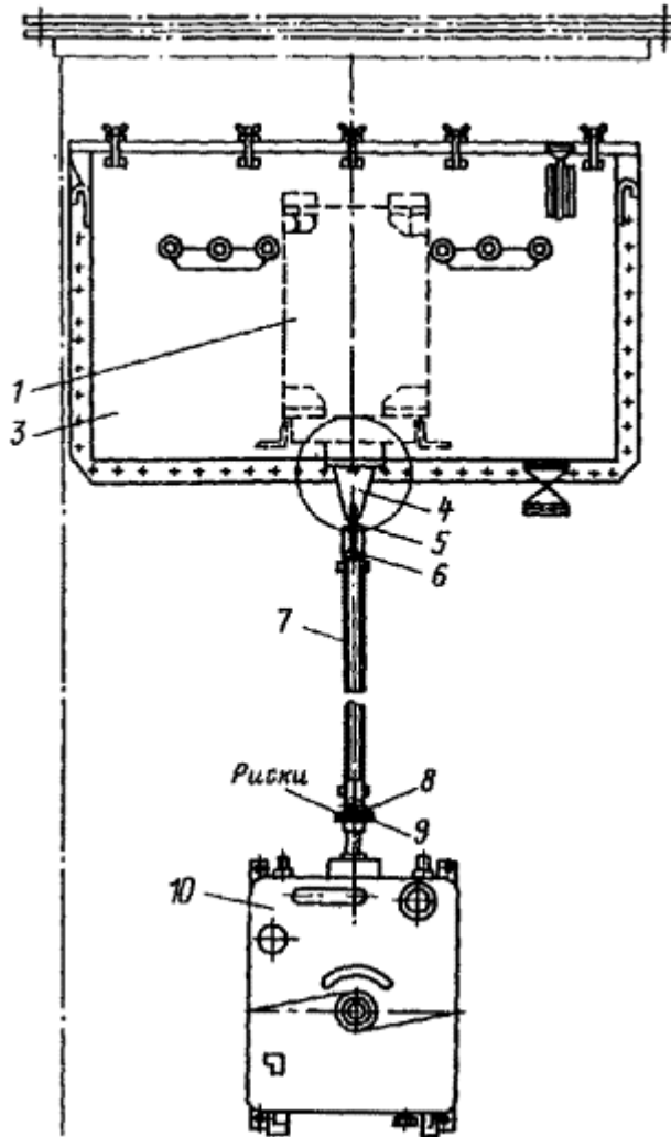
Рис. 15. Аппаратура для регулирования напряжения под нагрузкой.
