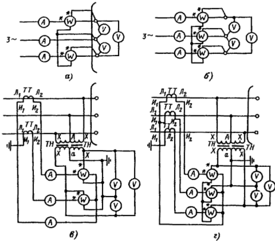
Рис. 24. Схемы включения приборов при прогреве трехфазных трансформаторов токами короткого замыкания.
