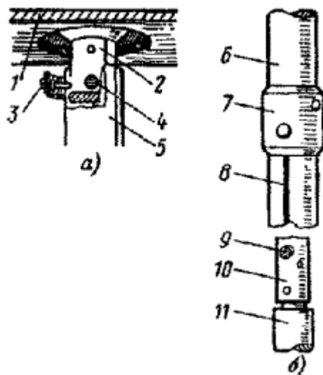
Рис. 13. Детали привода переключателя барабанного типа.
