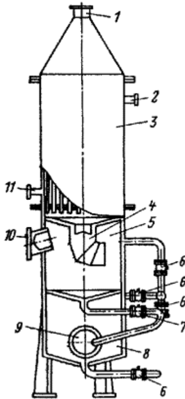
Рис. 30. Охладительная колонка.
