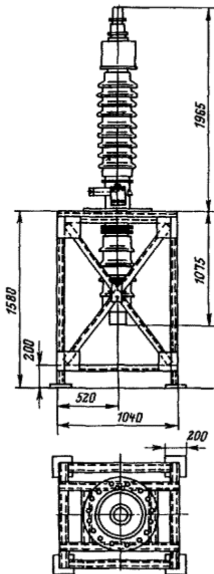
Рис. 2. Стойка для хранения ввода напряжением 110 кВ.
