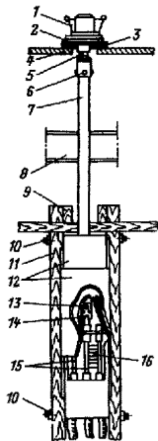
Рис. 12. Монтаж привода переключателя барабанного типа.
