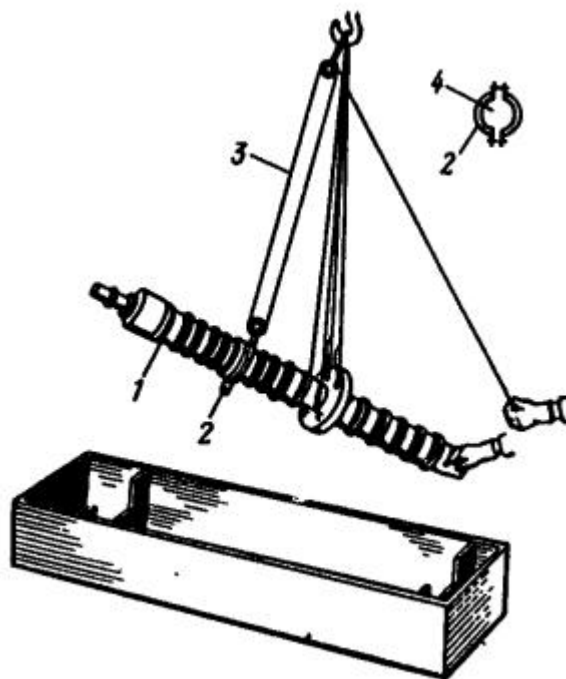
Рис. 3. Подъем маслонаполненного ввода напряжением 110 кВ из упаковки.
