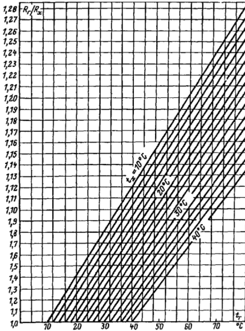
Рис. 27. Номограмма для определения температуры обмотки нагретого трансформатора постоянным током по отношению омических сопротивлений \frac{R_r}{R_x} .
